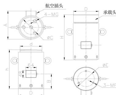
5000-50000kN
