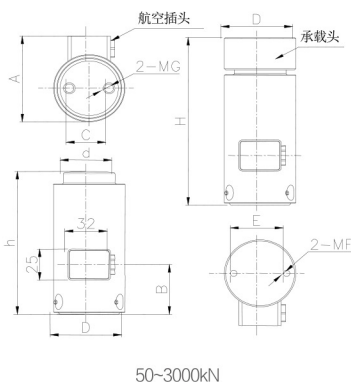
50-3000kN
